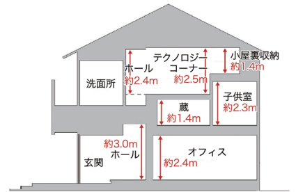
断面図(南)
