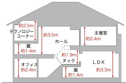
断面図(西)
