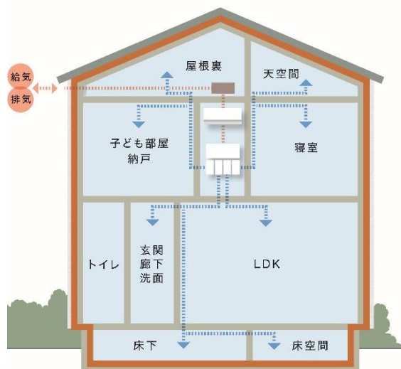
家をまるごと屋根裏から床下まで包みこむ 断熱区画と空調範囲
