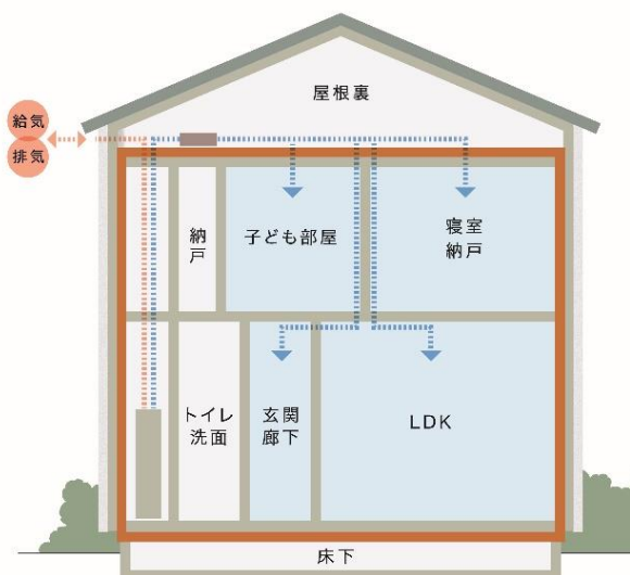
居室空間のみの 断熱区画と空調範囲
